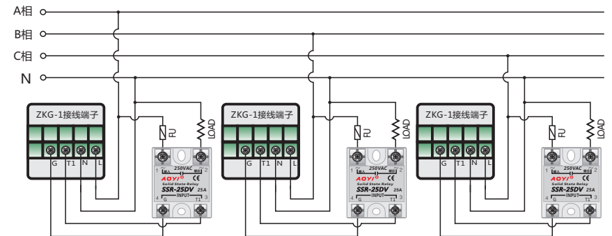
ZKG-1调整器配合SSR-DV模块三相接线图
